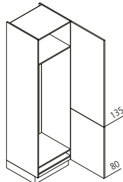
GKG Geräteschrank für Kühl- Gefrierkombination / Nische 159 cm ↔ 60 ↑ 215 ↶ 60
