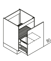
SABD Spülenunterschrank mit Abfalltrennsystem ↔ 45/50/60 ↑ 80 ↘ 60
