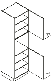
GB Geräteschrank für Backofen oder Mikrowelle ↔ 60 ↑ 215 ↶ 60
