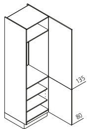
GK Geräteschrank für Kühlschrank / Nische 102,5 cm ↔ 60 ↑ 215 ↶ 60
