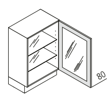
UDDDN Unterschrank mit Glastür DN ↔ 40/45/50/60 ↑ 80 ↘ 39
