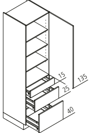
VAK Vorratsschrank ↔ 30/40/45/50/60 ↑ 215 ↶ 60/50
