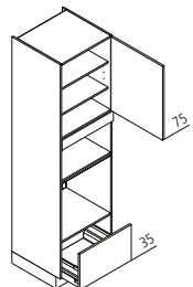
GBBA Geräteschrank für Backofen und Mikrowelle ↔ 60 ↑ 215 ↶ 60
