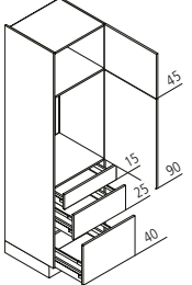
GKAK Geräteschrank für Kühlschrank / Nische 88 cm ↔ 60 ↑ 215 ↶ 60
