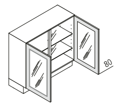
UDDDN Unterschrank mit Glastür DN ↔ 80/90/100/120 ↑ 80 ↘ 39
