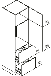
GKZ Geräteschrank für Kühlschrank / Nische 88 cm ↔ 60 ↑ 215 ↶ 60
