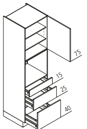
GBAK Geräteschrank für Backofen oder Mikrowelle ↔ 60 ↑ 215 ↶ 60
