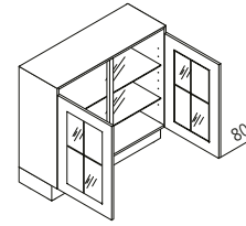
UDDVSP Unterschrank mit Glastür (programmabhängig) ↔ 80/90/100/120 ↑ 80 ↘ 60/39
