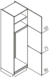
GK Geräteschrank für Kühlschrank / Nische 144 cm ↔ 60 ↑ 215 ↶ 60
