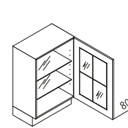
UDDVSP Unterschrank mit Glastür (programmabhängig) ↔ 40/45/50/60 ↑ 80 ↘ 60/39
