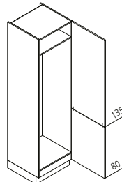
GK Geräteschrank für Kühlschrank / Nische 178 cm ↔ 60 ↑ 215 ↶ 60
