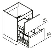
SUZ Spülenschränke mit Abfalltrennsystem ↔ 60/80/90/100/120 ↑ 80 ↘ 60
