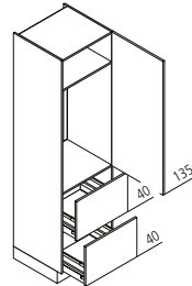
GKZ Geräteschrank für Kühlschrank / Nische 102,5 cm ↔ 60 ↑ 215 ↶ 60
