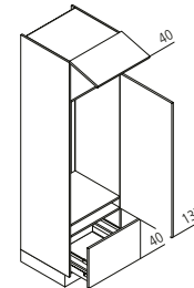
GKA Geräteschrank / Nische 102,5 cm ↔ 60 ↑ 215 ↶ 60
