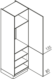
GK Geräteschrank für Kühlschrank / Nische 88 cm ↔ 60 ↑ 215 ↶ 60
