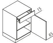
U Unterschrank
