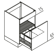
SAB Spülenunterschrank mit Abfalltrennsystem ↔ 45/50/60 ↑ 80 ↘ 60
