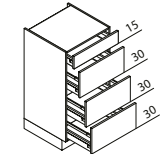
VAK Vorratsschrank ↔ 30/40/45/50/60 ↑ 105 ↱ 60/50
