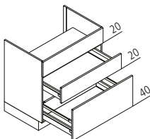
KAS Kochstellenschrank für Muldenlüfter
