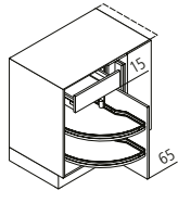
UEA Unterschränke-Ecke ↔ 110/115/125 ↑ 80 ↘ 60
