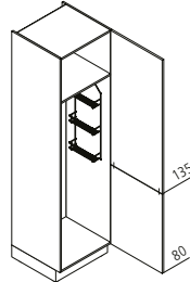
VB Besenschrank ↔ 30/40/45/50/60 ↑ 215 ↶ 60/50
