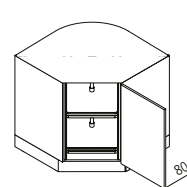
UETD Unterschränke-Ecke ↔ 90 ↑ 80 ↘ 60/50/39
