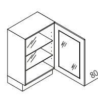
UDDV Unterschrank mit Glastür (programmabhängig) ↔ 40/45/50/60 ↑ 80 ↘ 60/39
