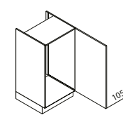
GK Geräteschrank für Kühlschrank / Nische 102,5 cm ↔ 60 ↑ 105 ↱ 60
