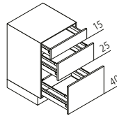
UAK Auszugsschrank
