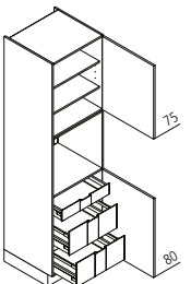
GBI Geräteschrank für Backofen oder Mikrowelle ↔ 60 ↑ 215 ↶ 60
