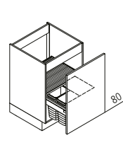
SABHD Spülenunterschrank mit hängendem Abfalltrennsystem ↔ 45/50/60 ↑ 80 ↘ 60
