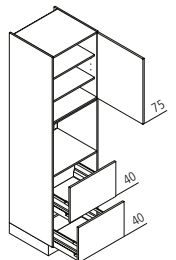
GBZ Geräteschrank für Backofen oder Mikrowelle ↔ 60 ↑ 215 ↶ 60
