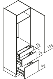
GKAK Geräteschrank für Kühlschrank / Nische 102,5 cm ↔ 60 ↑ 215 ↶ 60
