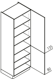
VT Vorratsschrank ↔ 30/40/45/50/60 ↑ 215 ↶ 60/50/39
