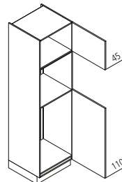
GKB Geräteschrank für Backofen, Kühlschrank / Nische 102,5 cm ↔ 60 ↑ 215 ↶ 60
