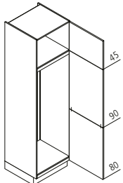
GK Geräteschrank für Kühlschrank / Nische 159 cm ↔ 60 ↑ 215 ↶ 60
