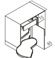
UELA Unterschränke-Ecke „Le Mans“ ↔ 110/115/125 ↑ 80 ↘ 60
